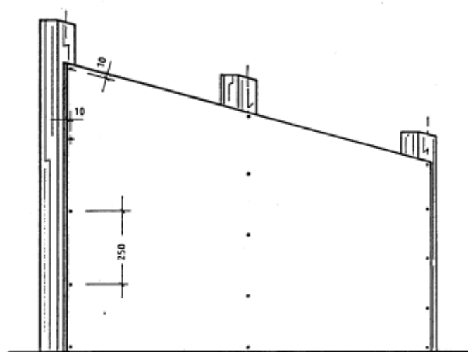
Figure 2 - Vissage sur ossature bois ou métal
